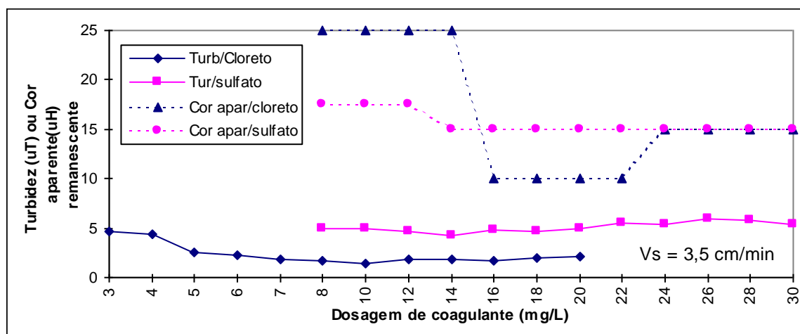
Figura 1: Turbidez remanescente ou cor aparente remanescente em função da dosagem de coagulante-Água tipo A, ETA-Morrinhos.
