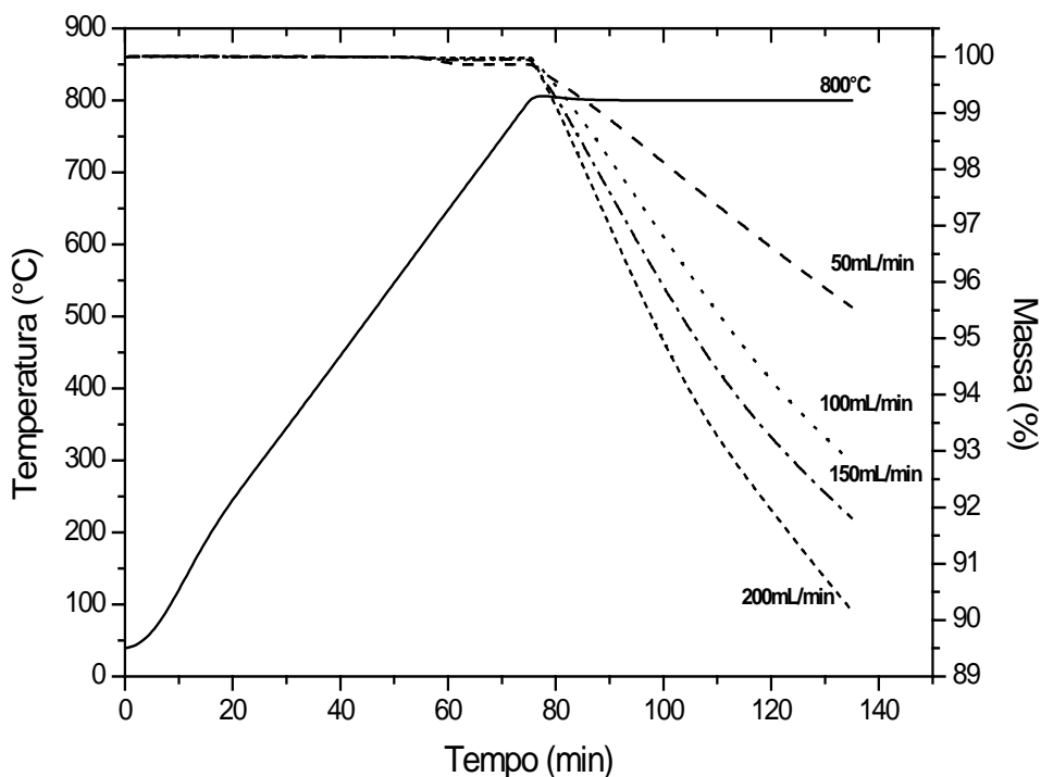
Figura 2: Curvas de análise termogravimétrica com isoterma de 800 °C, durante 1h em diferentes fluxos.
