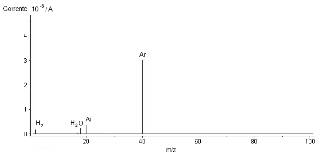
Figura 6: Espectro de massa das espécies da redução no fluxo de 200 ml/min.
