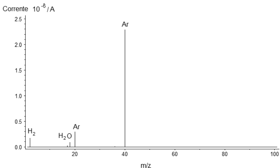
Figura 3: Espectro de massa das espécies da redução no fluxo de 100 ml/min.
