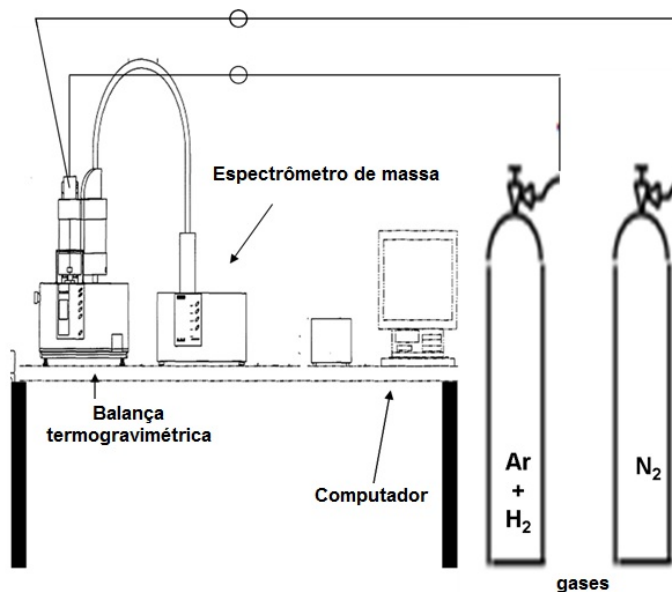
Figura 1: Fluxograma do aparato experimental.
