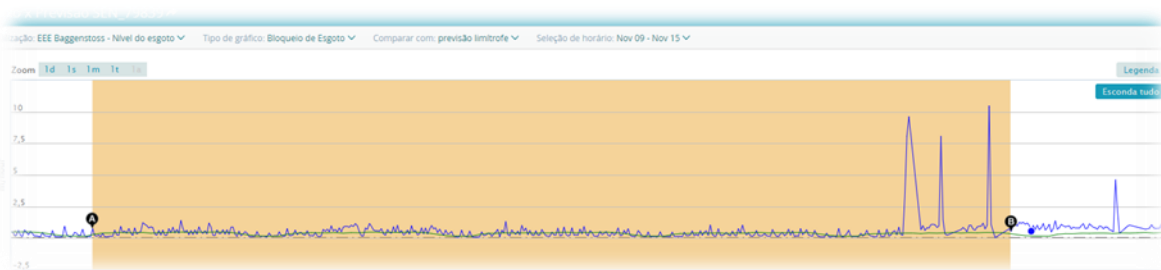
Figura 8 – Evento de nível de esgoto (obstrução identificada)
