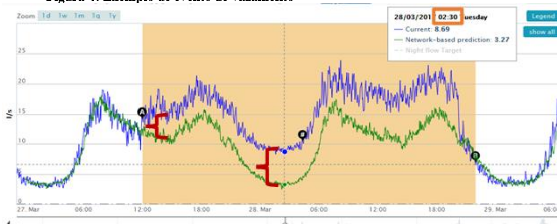
Figura 4: Exemplo de evento de vazamento
