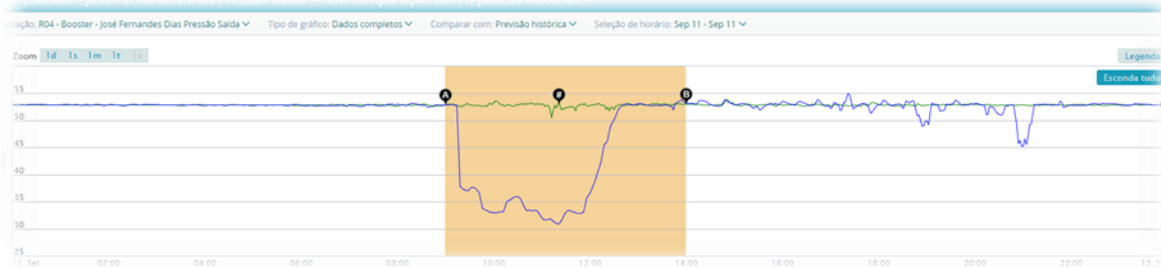
Figura 7 – Evento de pressão (vazamento de ramal identificado)
