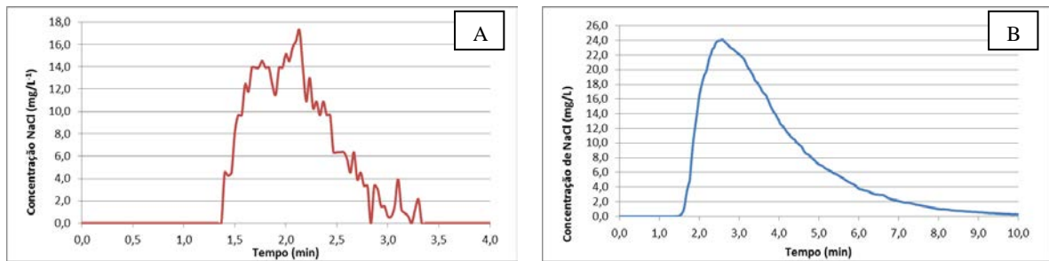
Figura 3: Ensaios hidrodinâmicos: A – Insatisfatório; B – Satisfatório.
