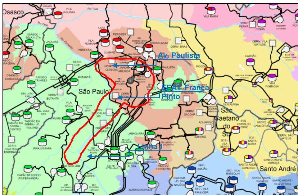
Figura 3 – Esquema hidráulico do SAM com destaque a região da Avenida Paulista.
