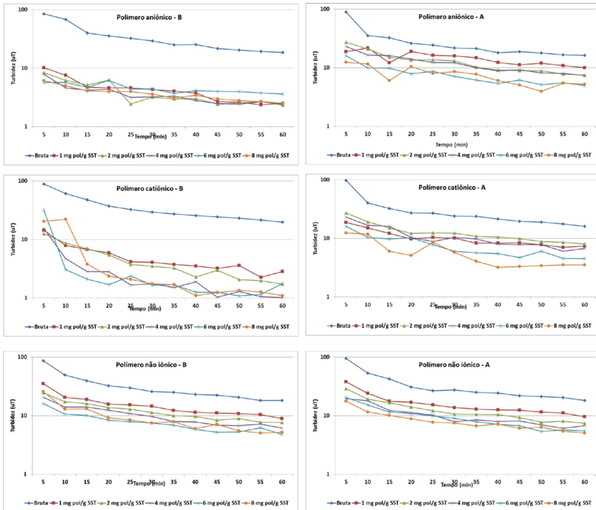
Figura 2: Turbidez do sobrenadante (água clarificada) nos ensaios de clarificação e adensamento por gravidade
