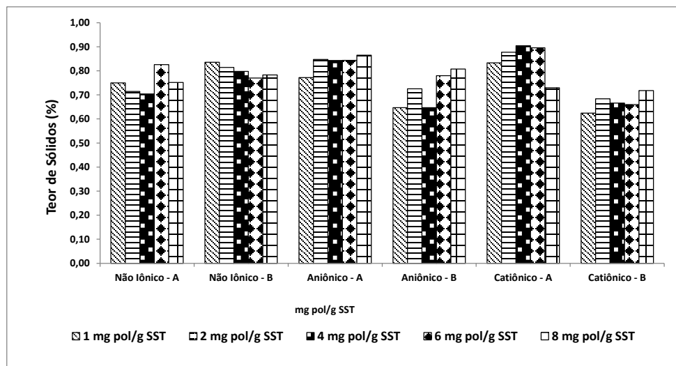
Figura 3: Teor de sólidos no lodo final nos ensaios de clarificação e adensamento por gravidade
