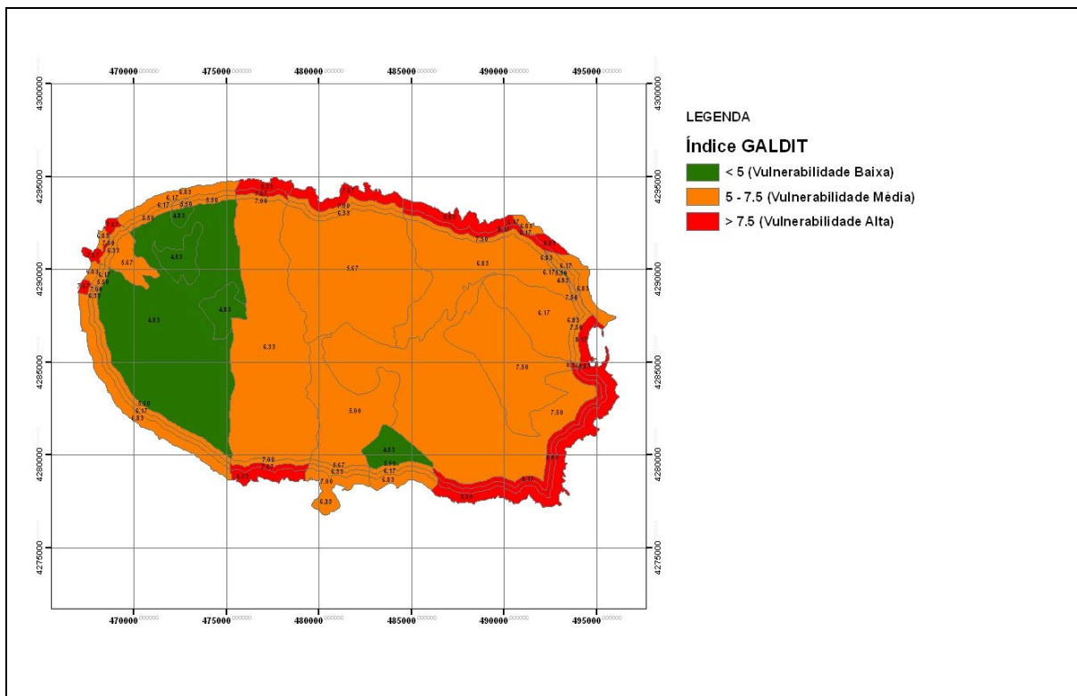
Figura 1: Índice GALDIT para os aquíferos da ilha Terceira (Açores).
